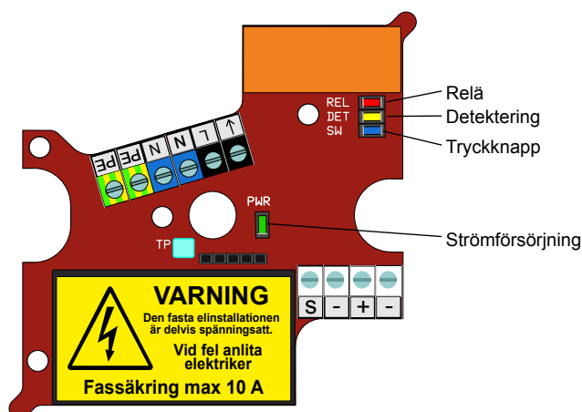
Kretskort i strömförsörjningsmodul PS-230
