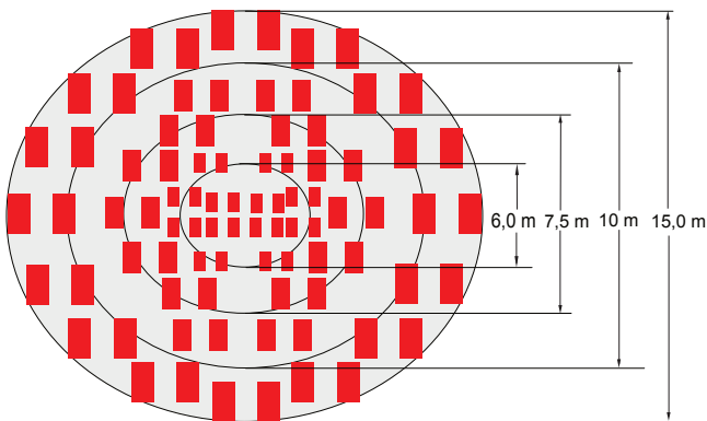
Ovanifrån
